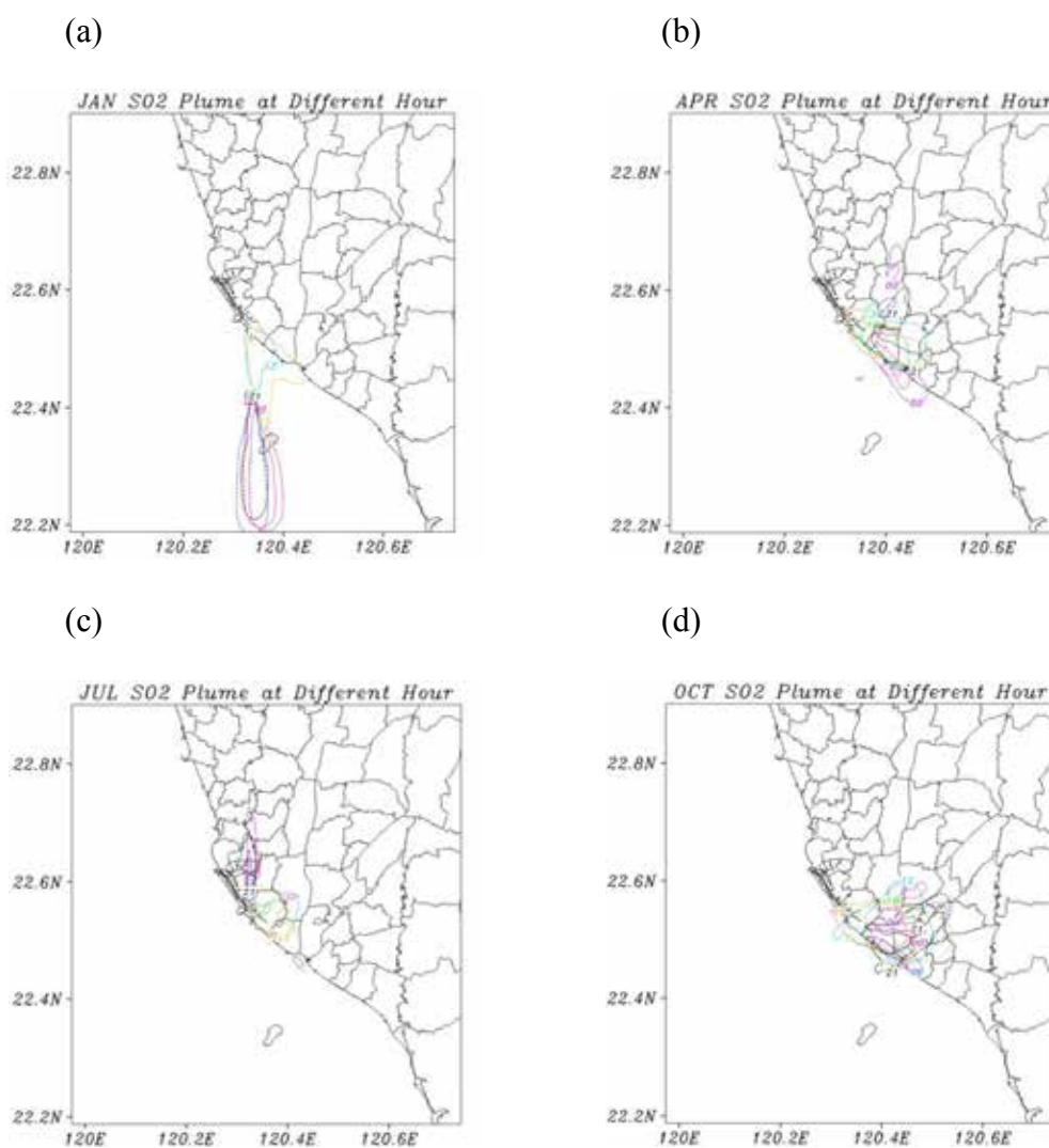
圖 5. 1 月、4 月、7 月及 10 月不同時間點污染物濃度分布圖，等值線上的數字為時間點，其中(a)為 1 月，(b)為 4 月，(c)為 7 月，(d)為 10 月
