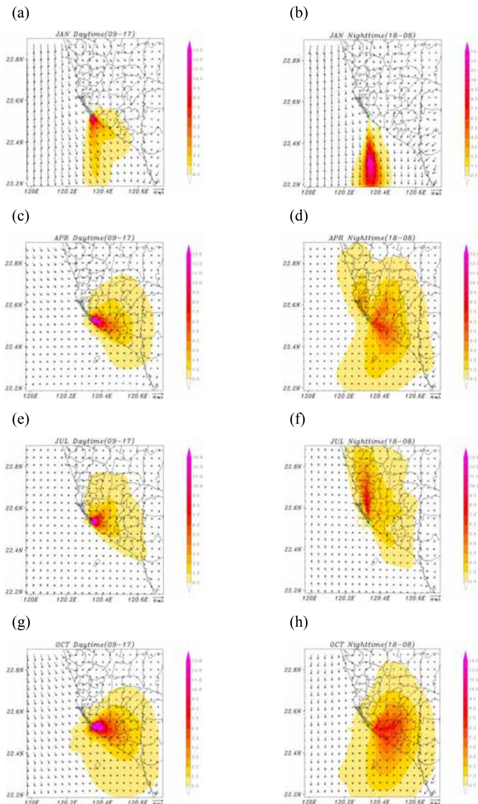
圖 4.日、夜污染物濃度（色階）分布與風場（向量）合成圖，其中(a)為 1 月日間平均，(b)為 1 月夜間平均，(c)為 4 月日間平均，(d)為 4 月夜間平均，(e)為 7 月日間平均，(f)為 7 月夜間平均，(g)為 10 月日間平均，(h)為 10 月夜間平均
