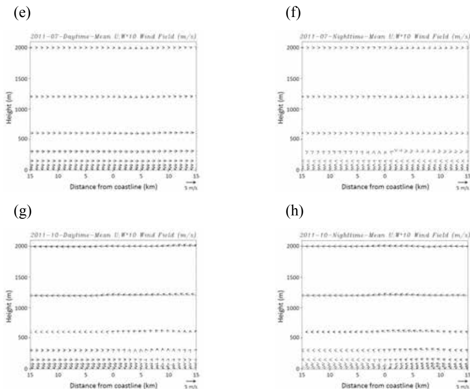
圖 6. 2011 年 1 月、4 月、7 月及 10 月日、夜海岸區域東西向一垂直月平均風場，其中(a)為 1 月日間平均，(b)為 1 月夜間平均，(c)為 4 月日間平均，(d)為 4 月夜間平均，(e)為 7 月日間平均，(f)為 7 月夜間平均，(g)為 10 月日間平均，(h)為 10 月夜間平均
