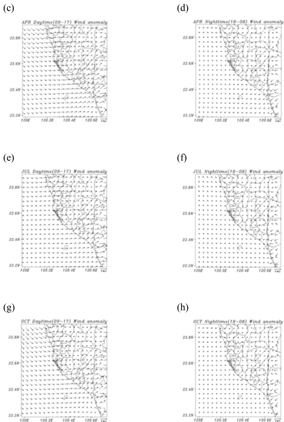
圖 7. 2011 年 1 月、4 月、7 月及 10 月日、夜風場距平，其中(a)為 1 月日間平均，(b)為 1 月夜間平均，(c)為 4 月日間平均，(d)為 4 月夜間平均，(e)為 7 月日間平均，(f)為 7 月夜間平均，(g)為 10 月日間平均，(h)為 10 月夜間平均
